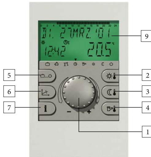
Gestore di zona VICTRIX 50
